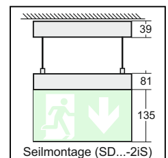
Seilmontage (SD...-2iS)
