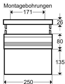
Pendelmontage mit Deckenbaldachinschiene:
