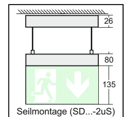
Seilmontage (SD...-2uS)
