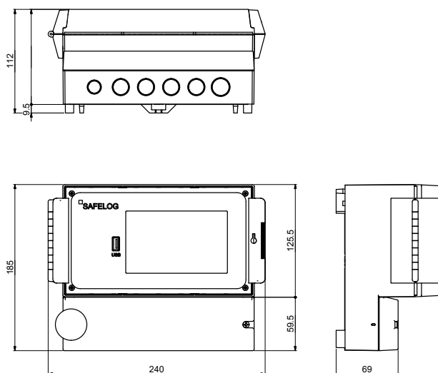
Abb. 1: Maßzeichnung SAFELOG
