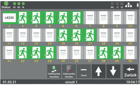
Abb. 68: „Übersicht Auswahl Verbraucher“
