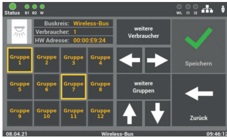
Abb. 80: Maske „Zuordnungen – Gruppen“
