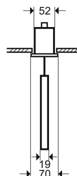
mind. 8 mm Deckenplattenstärke
