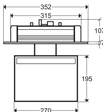
Deckeneinbaumontage (SE): (Deckenausschnitt: 315 x 55 mm)
