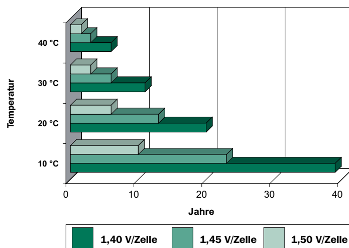
Wartungsintervall für grid | power FNC-VR - L-Typen Jahre bei Temperatur und Ladespannung
