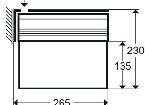
2 Kabeleinführungen, hintereinander
