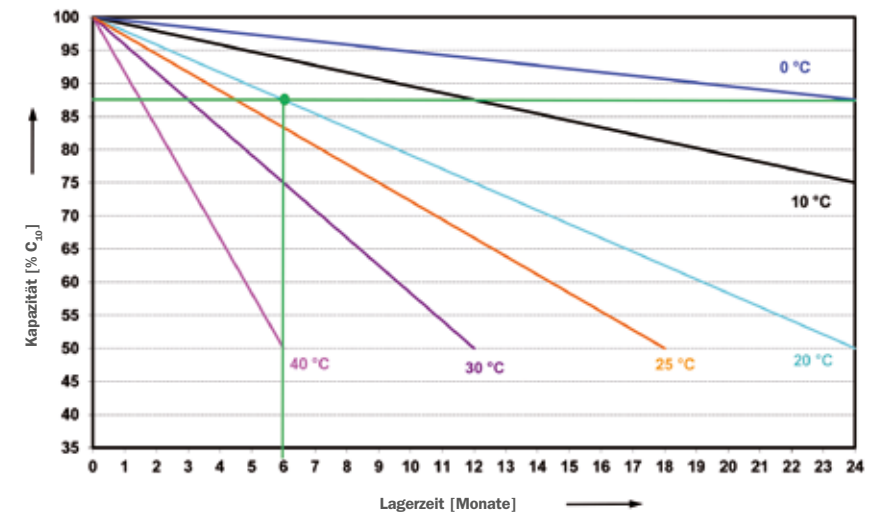
Abb. 4-1: Kapazität über Lagerzeit
