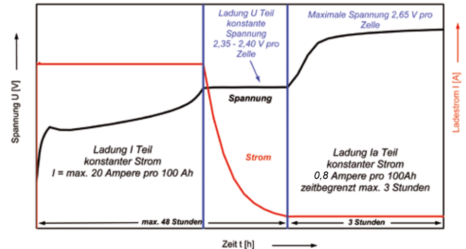
Abb. 9-2: Kennlinie IUla
