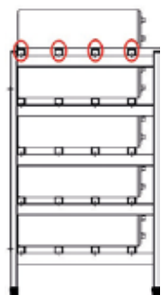
Zellen 12 OPzV 1500 Ah bis 24 OPzV 3000 Ah
