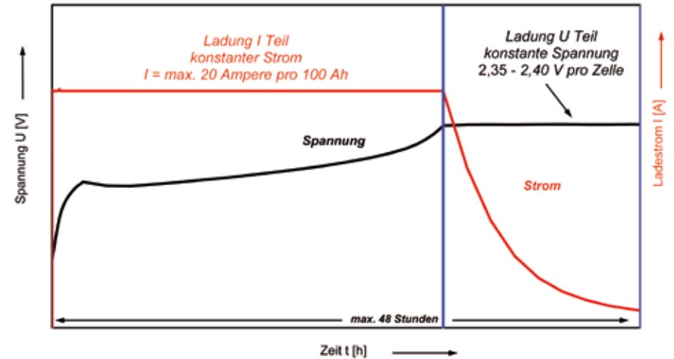
Abb. 9-1: Kennlinie IU
