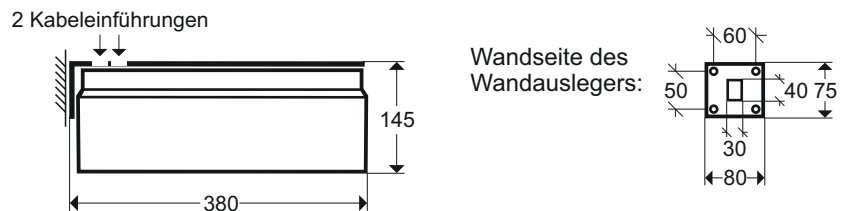
Wandauslegermontage (K21...-WA):
