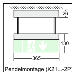
Pendelmontage (K21...-2P)
