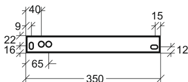
Deckenmontage, direkt (SD): (Ansicht von oben)
