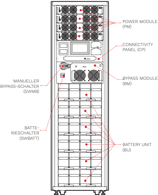
MPX 100 CBC MPX Combo Cabinet 15–60 kW oder 25–100 kW (Vorderseite)
