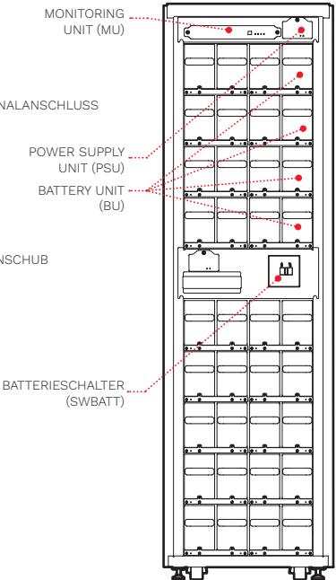
MPW 170 BTC MPW Batterieschrank (Vorderseite)
