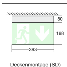
Deckenmontage (SD)
