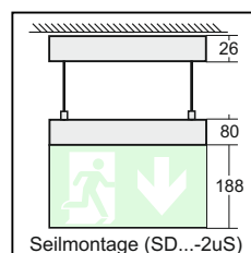
Seilmontage (SD...-2uS)
