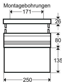
Pendelmontage mit Deckenbaldachinschiene:
