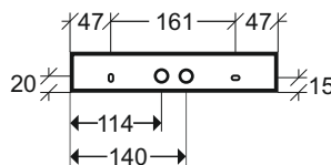
Deckenmontage, direkt (SD): (Ansicht von oben)
